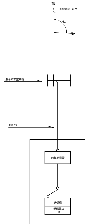
空中線系統図
