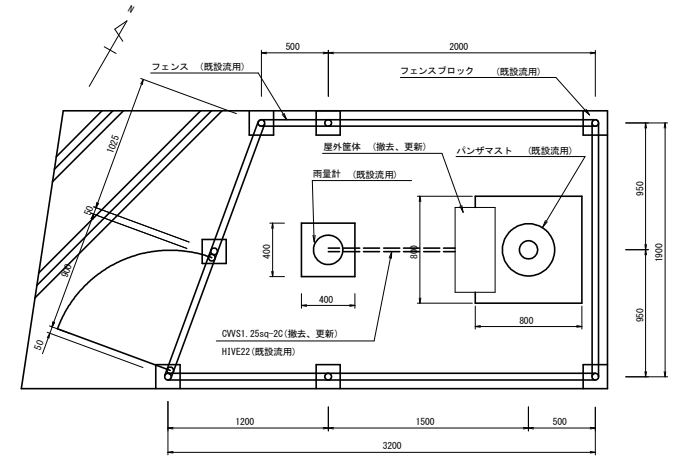
敷地平面図
