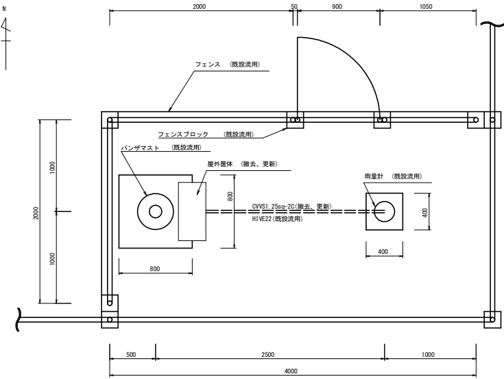
敷地平面図 (S=1/20)
