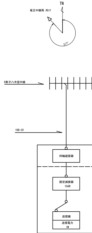
空中線系統図
