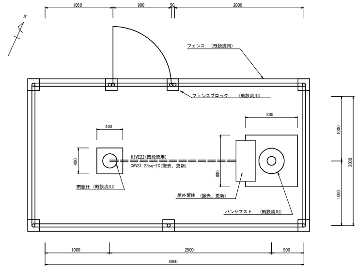
敷地平面図 (S=1/20)
