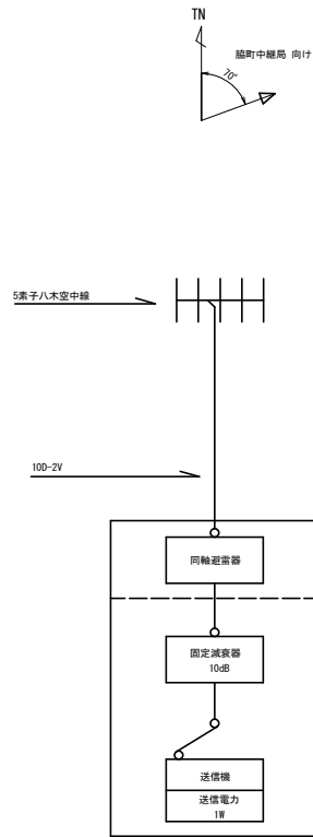
空中線系統図 (S=1/20)
