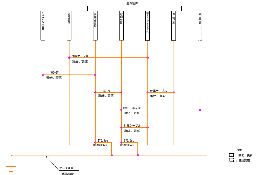
配線系統図
