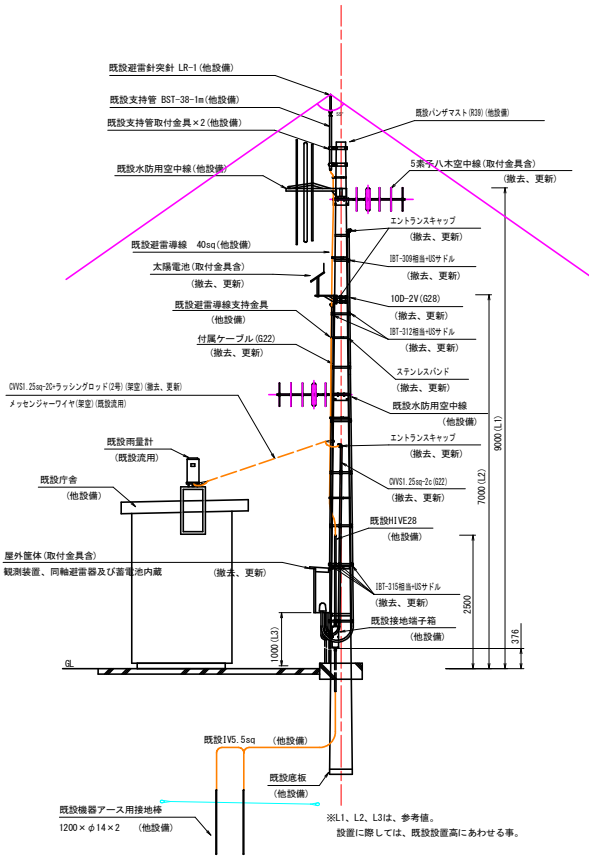
基本実装図(標準図)
