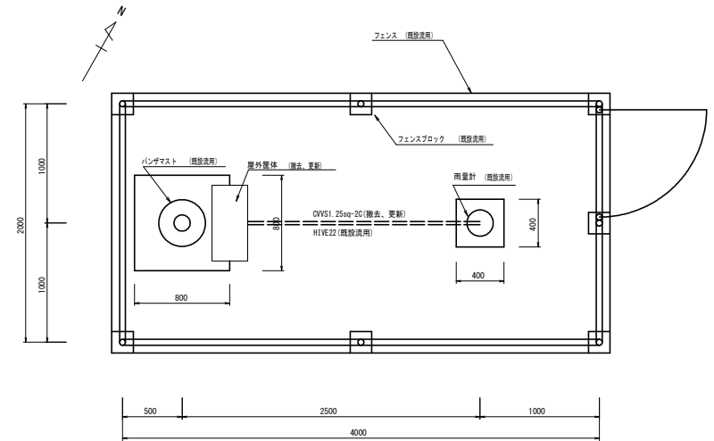
敷地平面図
